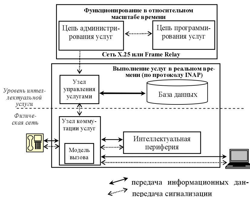
Рис. 1.25. Физическая архитектура интеллектуальной сети
