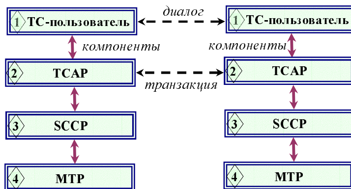
Рис. 1.22. Информационные элементы TCAP
