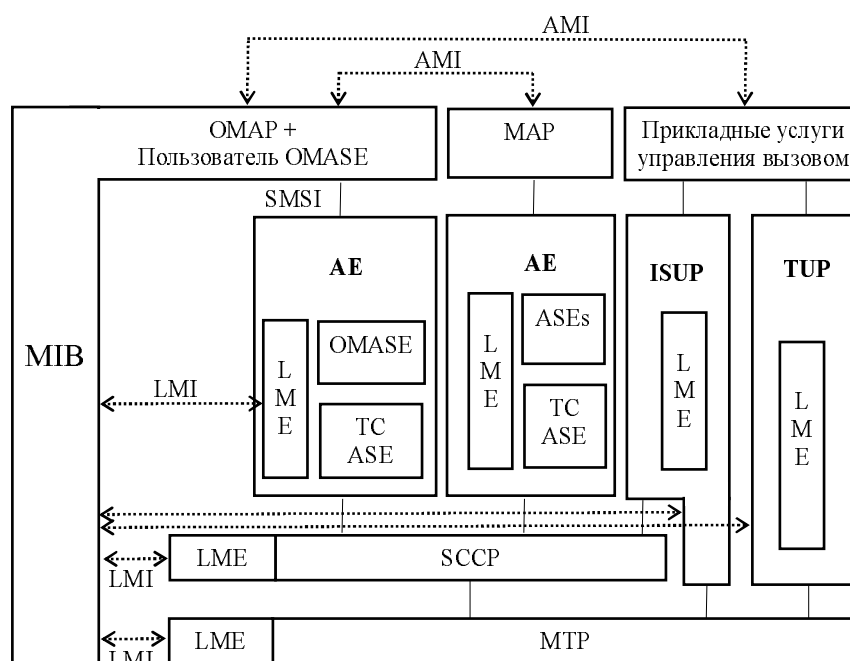
Рис. 1.29. Модель управления сетью ОКС № 7
