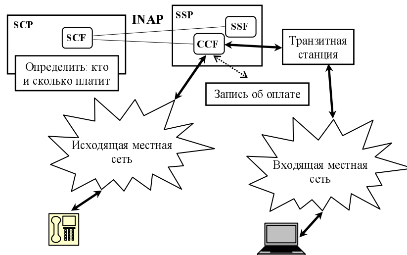
Рис. 1.26. Алгоритм предоставления интеллектуальной услуги «с дополнительной платой»
