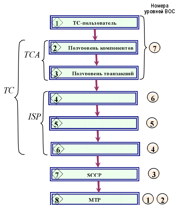
Рис. 1.21. Структура ТС и её положение в ОКС № 7
